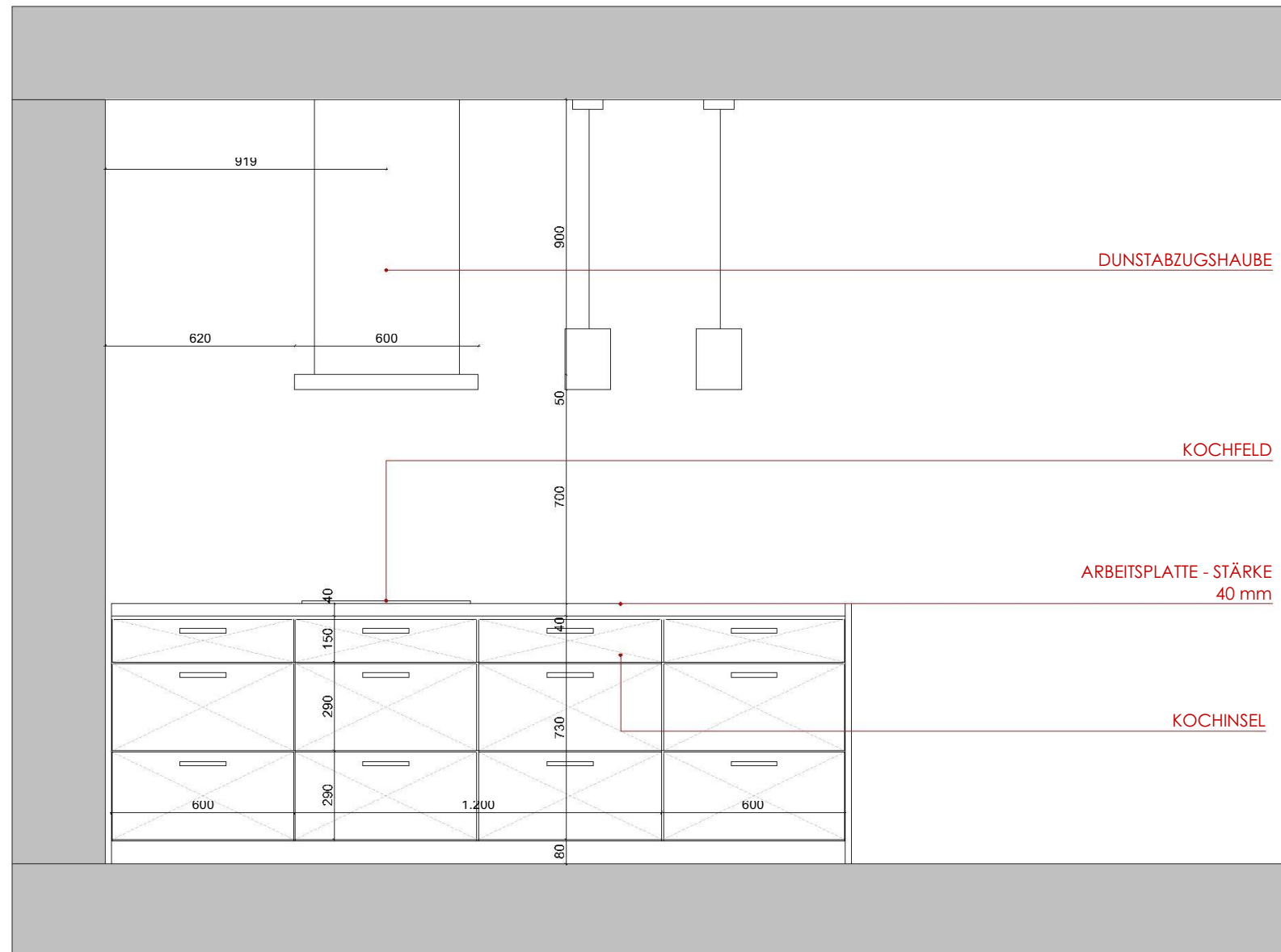
KUCHE SCHNITT 3
