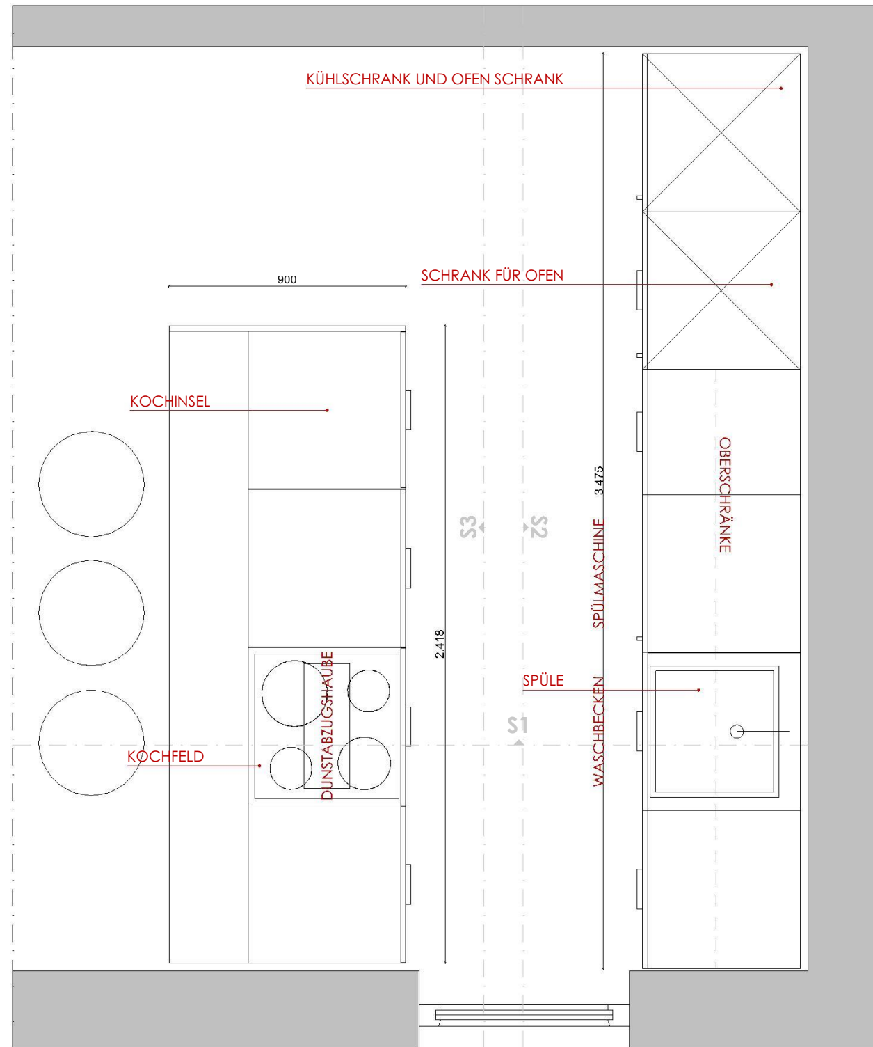
KUCHE GRUNDRISS
